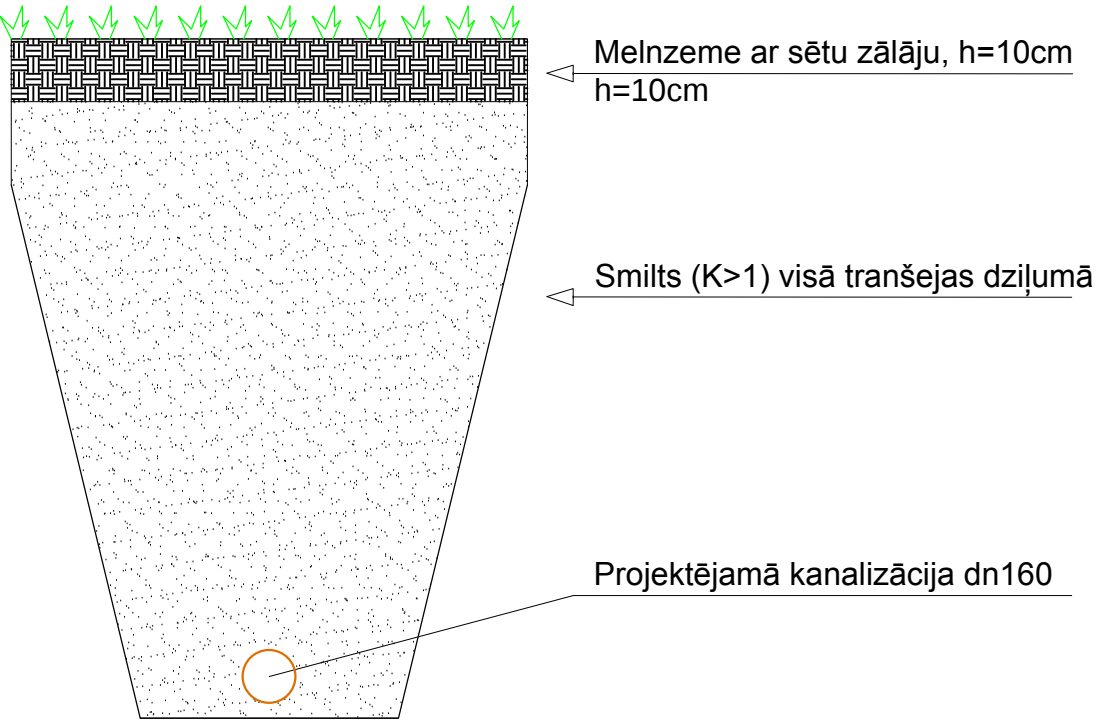
Zālāja atjaunošana izbūvējamā ūdensvada tranšejā
