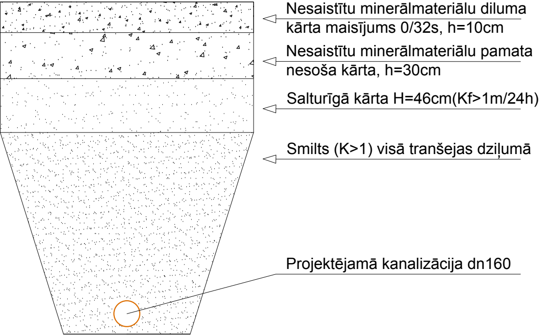
Ceļa (grants seguma) atjaunošana izbūvējamā ūdensvada tranšejā
